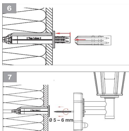
application B : montage élément de construction
