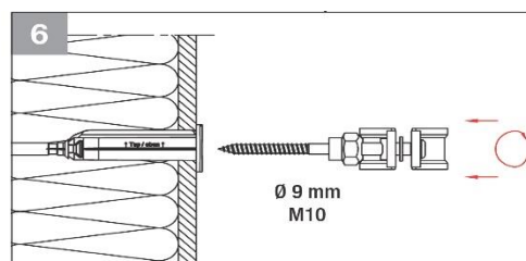
application A : montage élément de construction
