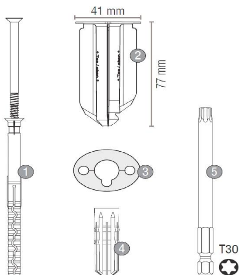
1 - 4: Onderdelen van de StoFix Iso-Dart
