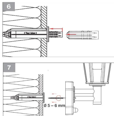
Toepassing A: Montage bouwdeel
